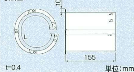
寸法図
